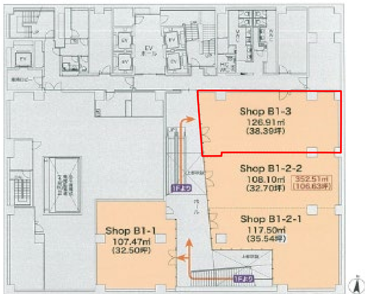
地下1階平面図 店舗天井高/3.000m
